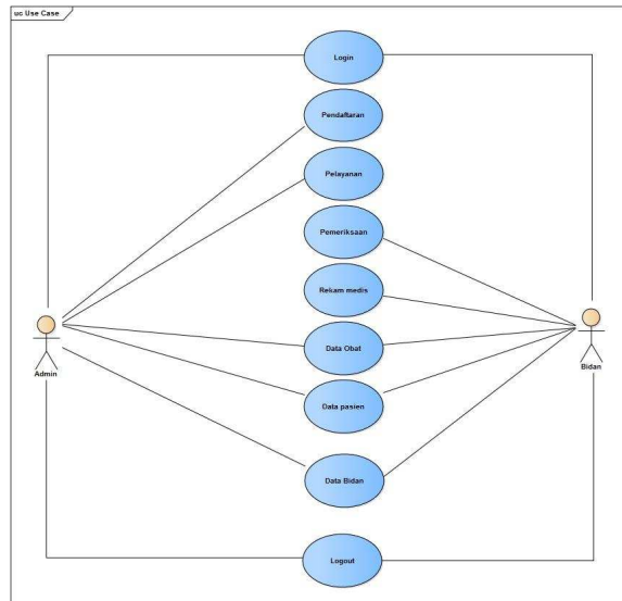
Gambar IV.1 Rancangan Use Case Diagram
