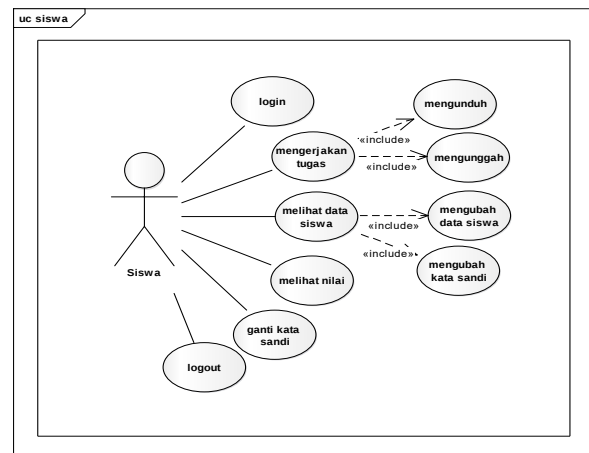
Gambar 2. Use Case Halaman Siswa
